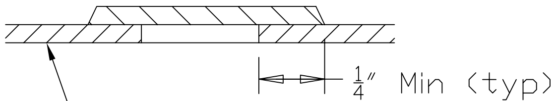
Amer-Plate Sheet Section A-A
